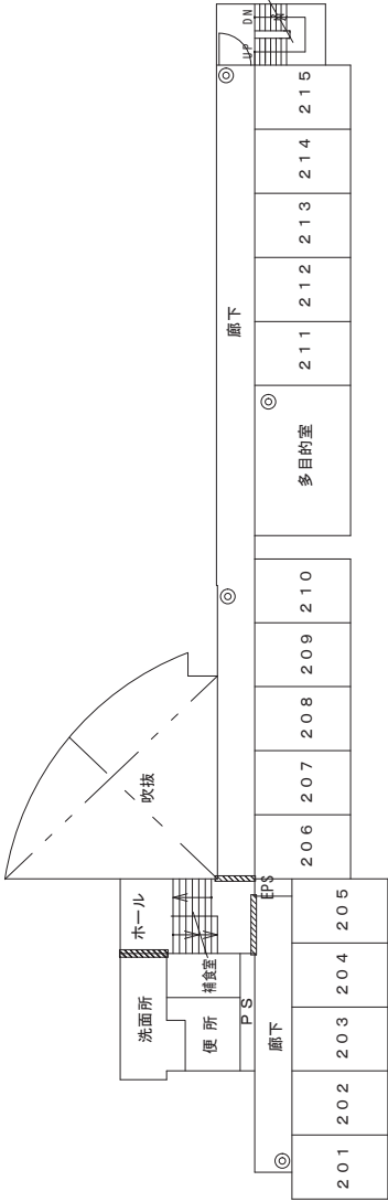
2階平面図
